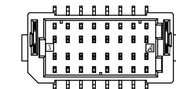
16~60PIN Housing有缺口示意图
