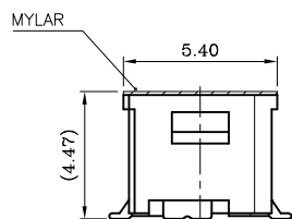
12 PIN - MYLAR
