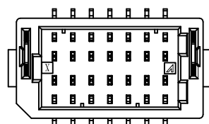
8~14PIN Housing無缺口示意图
